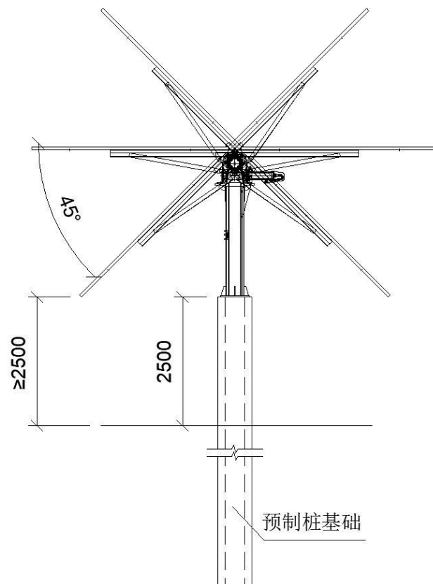
图 1-1 平单轴跟踪式光伏支架结构图
